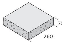
Krönplatta pelare
